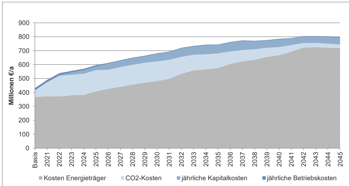
Abbildung 22: jährliche energiebezogene Kosten bis 2045 im Biogaspfad (Pfad 1) unter Annahme eines Fremdbezugs von Biomethan
