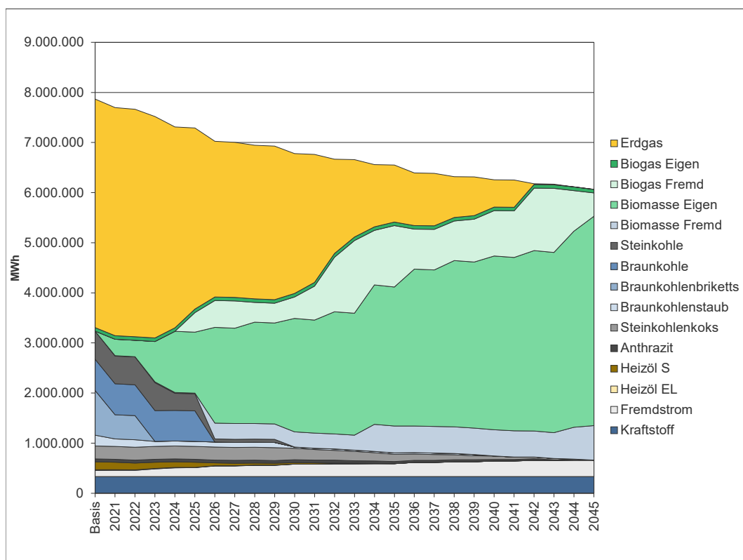
Abbildung 24: Entwicklung des Energieträgereinsatzes bis 2045 im Biomassepfad (Pfad 2)
