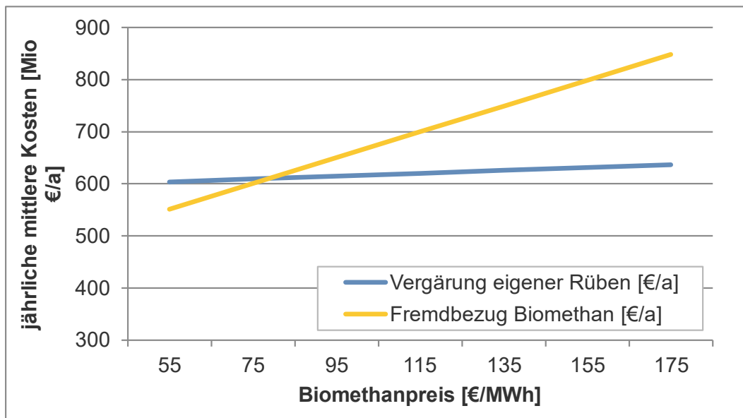
Abbildung 23: Sensitivitätsbetrachtung der mittleren jährlichen energiebezogenen Kosten abhängig von den Bezugskosten für Biomethan
