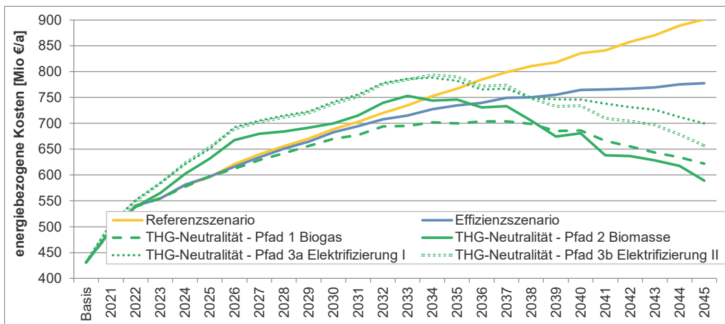
Abbildung 45: Energiebezogene Kosten aller Szenarien bei einem CO 2 -Preisfad bis 300 €/t im Jahr 2045
