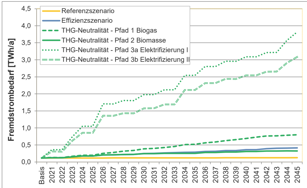
Abbildung 39: Entwicklung des Fremdstrombedarfs bis 2045 – Gegenüberstellung aller Szenarien
