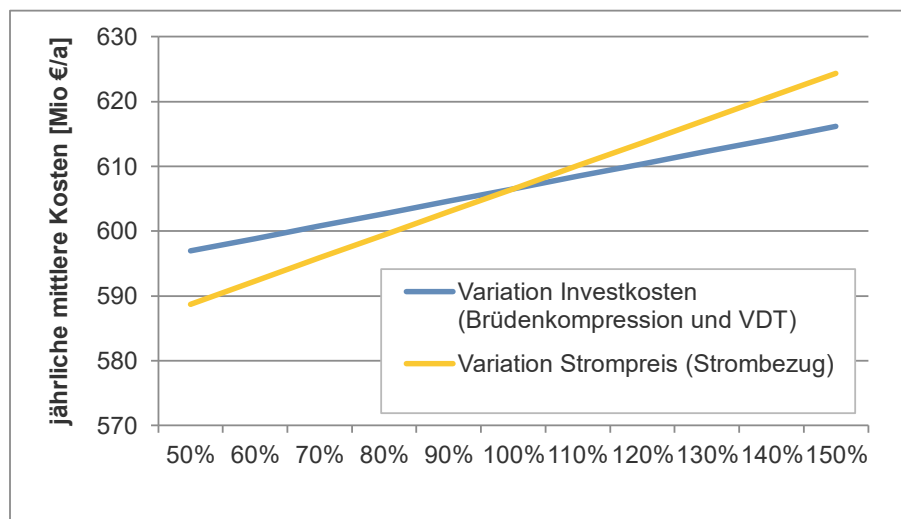
Abbildung 17: Sensitivitätsbetrachtung der mittleren jährlichen energiebezogenen Kosten abhängig von einer prozentualen Änderung der Investitionskosten bzw. des Strompreises
