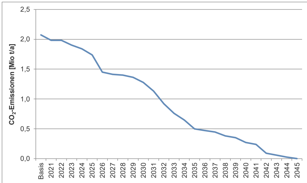
Abbildung 34: Entwicklung der CO 2 -Emissionen bis 2045 im Elektrifizierungspfad II (Pfad 3b)
