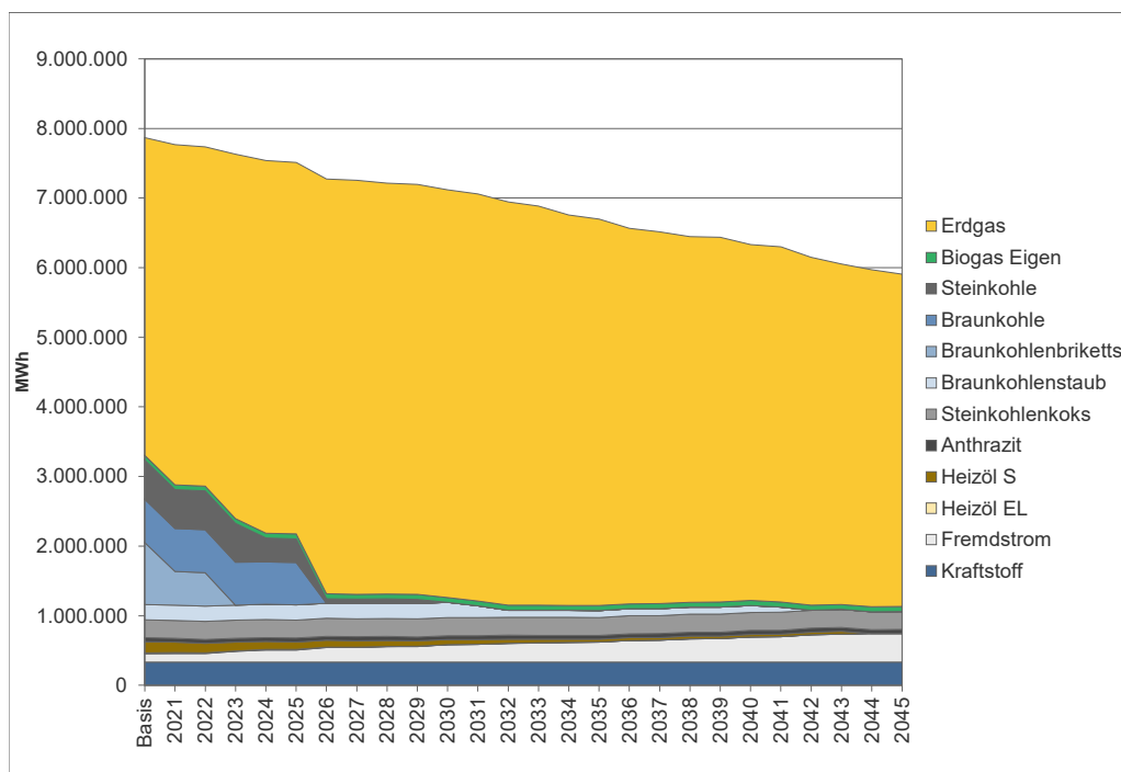
Abbildung 13: Entwicklung des Energieträgereinsatzes bis 2045 im Effizienzzenario
