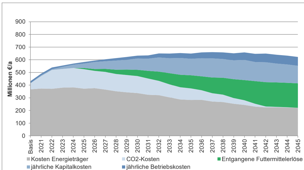
Abbildung 20: Entwicklung der jährlichen energiebezogenen Kosten bis 2045 im Biogaspfad (Pfad 1)
