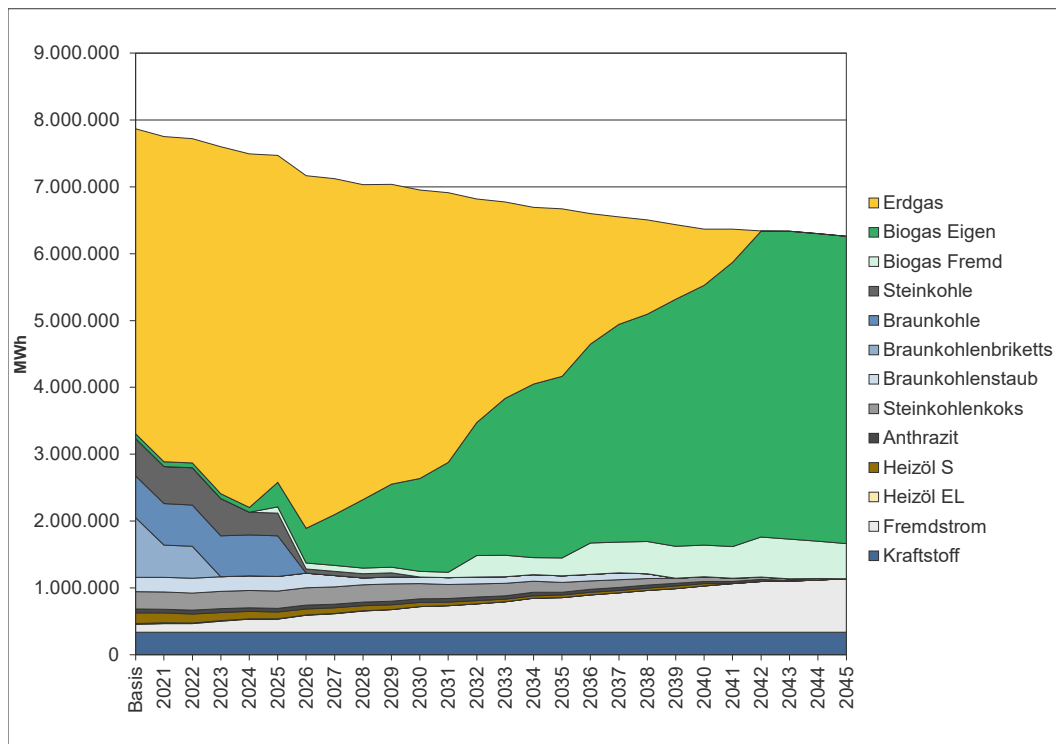
Abbildung 18: Entwicklung des Energieträgereinsatzes bis 2045 im Biogaspfad (Pfad 1)
