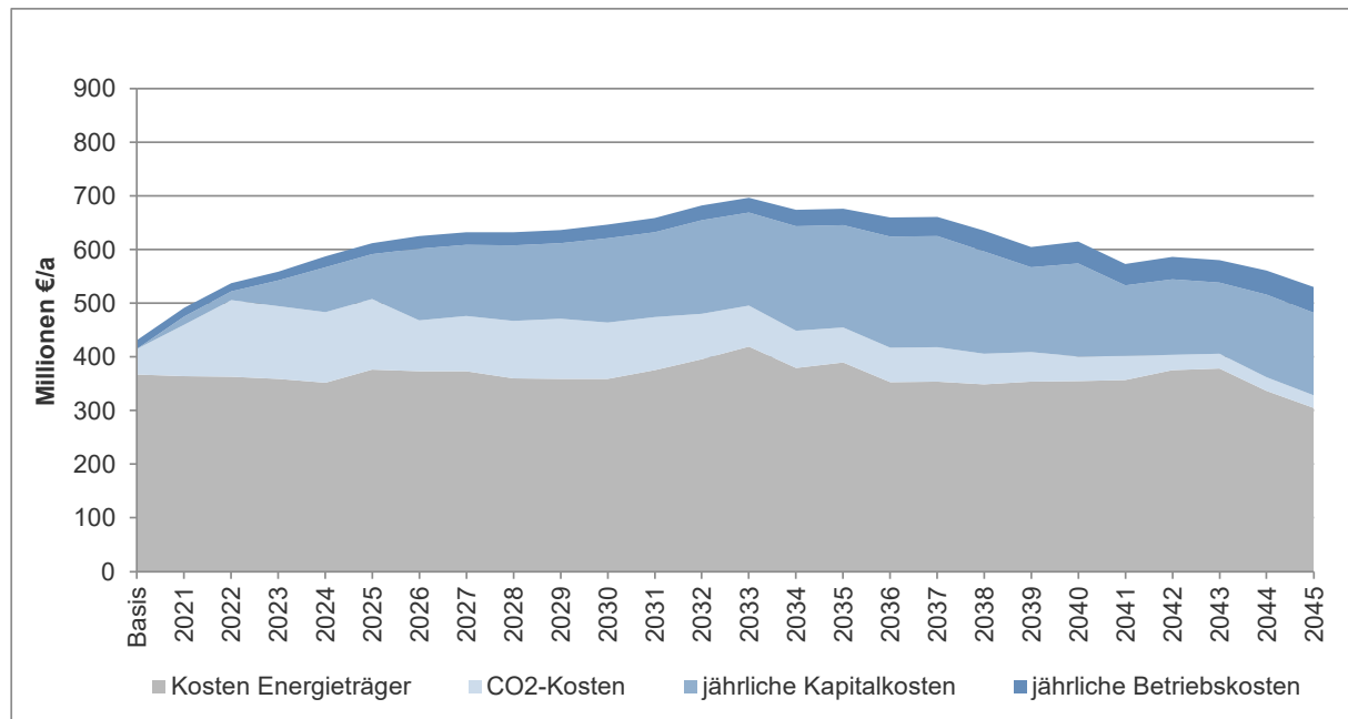
Abbildung 28: Entwicklung der jährlichen energiebezogenen Kosten bis 2045 im Biomassepfad (Pfad 2) unter Annahme eines Fremdbezugs von Biomasse
