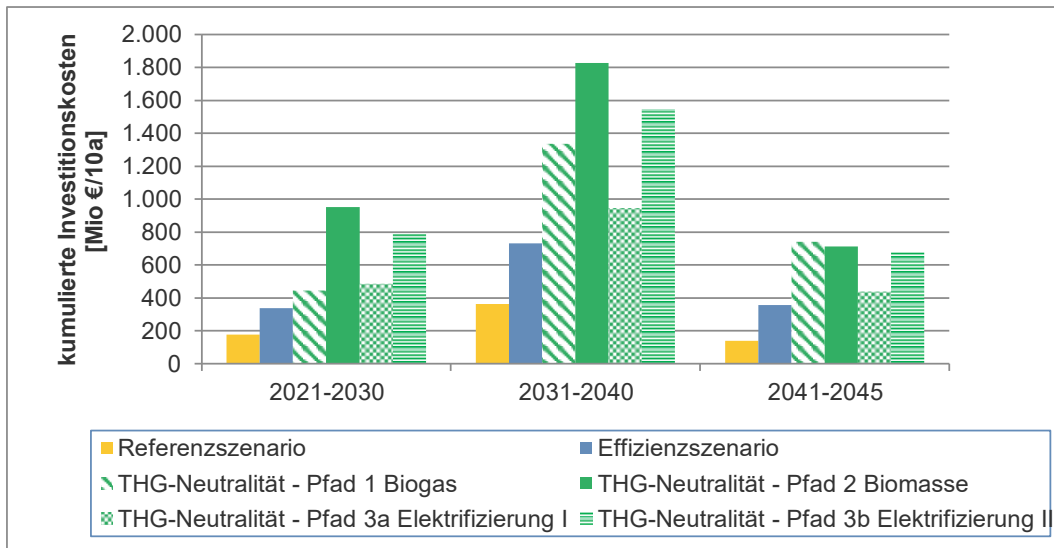
Abbildung 40: Darstellung der kumulierten Investitionskosten der betrachteten Szenarien
