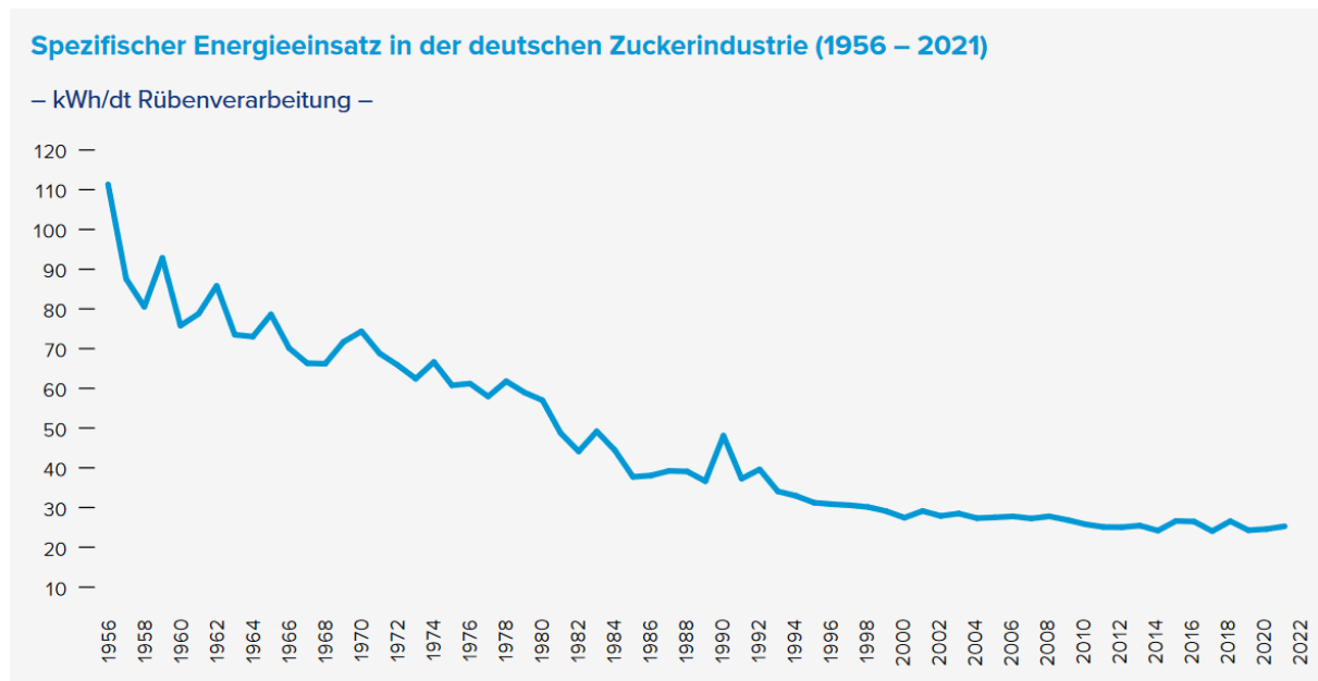
Abbildung 3: Entwicklung des spezifischen Energieeinsatzes in der deutschen Zuckerindustrie. Quelle: Jahresbericht 2022/2023 des Vereins der Zuckerindustrie e.V.
