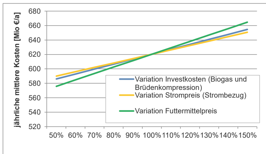
Abbildung 21: Sensitivitätsbetrachtung der mittleren jährlichen energiebezogenen Kosten abhängig von einer prozentualen Änderung der Investitionskosten bzw. des Strombezugspreises und des Futtermittelpreises
