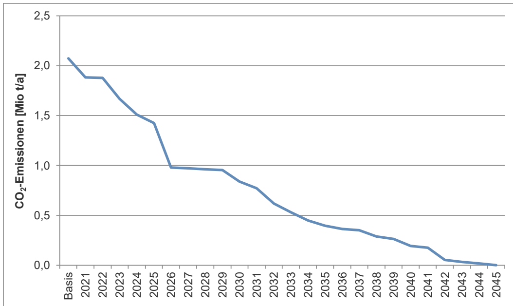
Abbildung 25: Entwicklung der CO 2 -Emissionen bis 2045 im Biomassepfad (Pfad 2)
