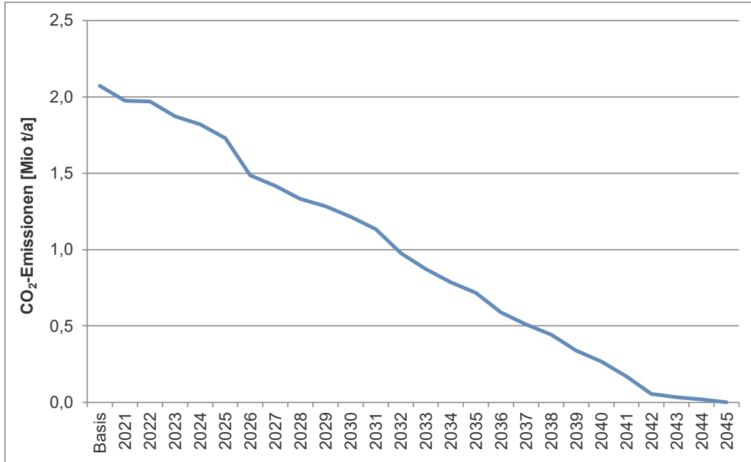
Abbildung 19: Entwicklung der CO 2 -Emissionen bis 2045 im Biogaspfad (Pfad 1)
