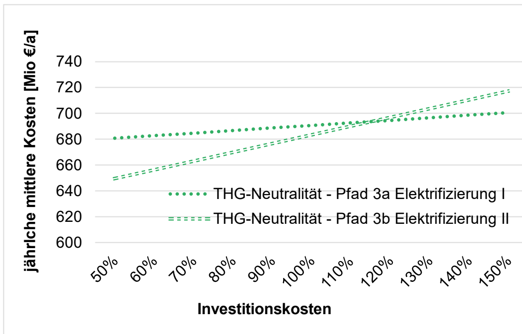
Abbildung 37: Sensitivitätsbetrachtung der mittleren jährlichen Kosten der beiden Elektrifizierungspfade abhängig von den Investitionskosten
