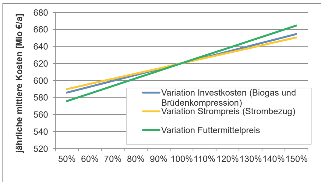
Abbildung 27: Sensitivitätsbetrachtung der mittleren jährlichen energiebezogenen Kosten abhängig von einer prozentualen Änderung der Investitionskosten bzw. des Strompreises und des Futtermittelpreises
