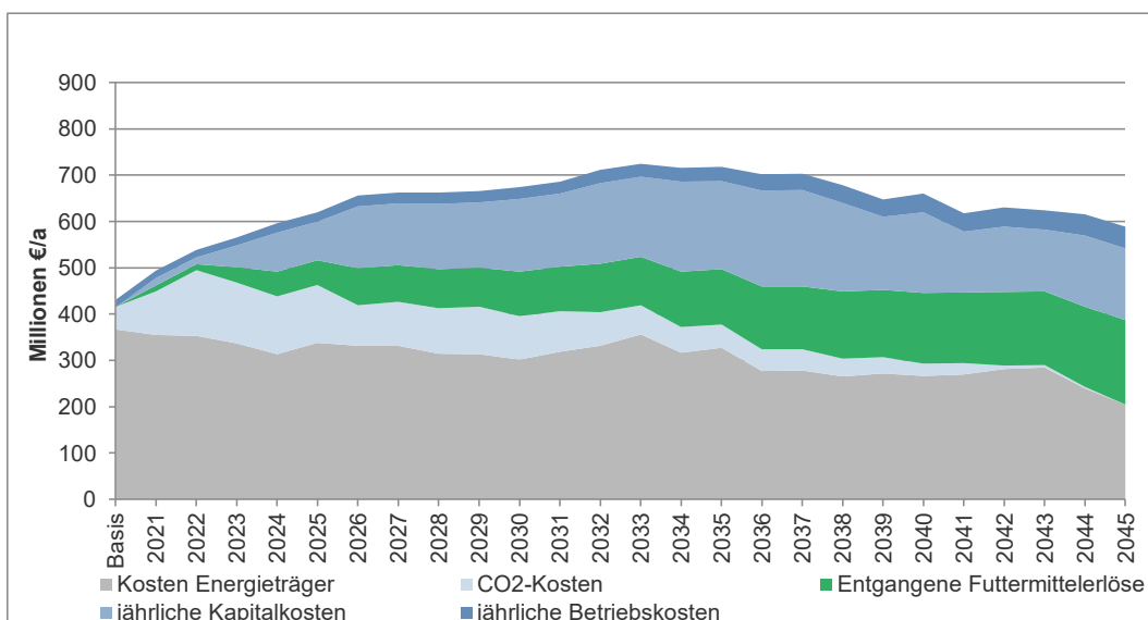
Abbildung 26: Entwicklung der jährlichen energiebezogenen Kosten bis 2045 im Biomassepfad (Pfad 2)
