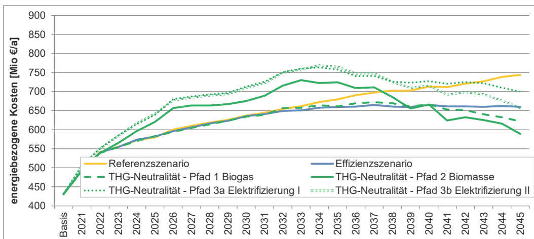
Abbildung 43 Energiebezogene Kosten aller Szenarien bei einem CO 2 -Preispfad bis 200 €/t im Jahr 2045
