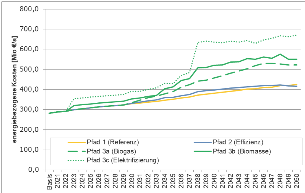
Abbildung 42 Entwicklung der energiebezogenen Kosten – Gegenüberstellung aller Pfade aus der Fassung von 2020
