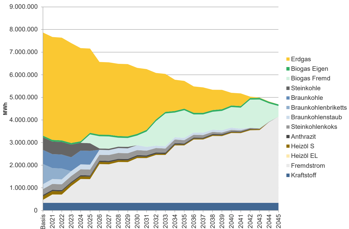
Abbildung 30: Entwicklung des Energieträgereinsatzes bis 2045 im Elektrifizierungspfad (Pfad 3a)
