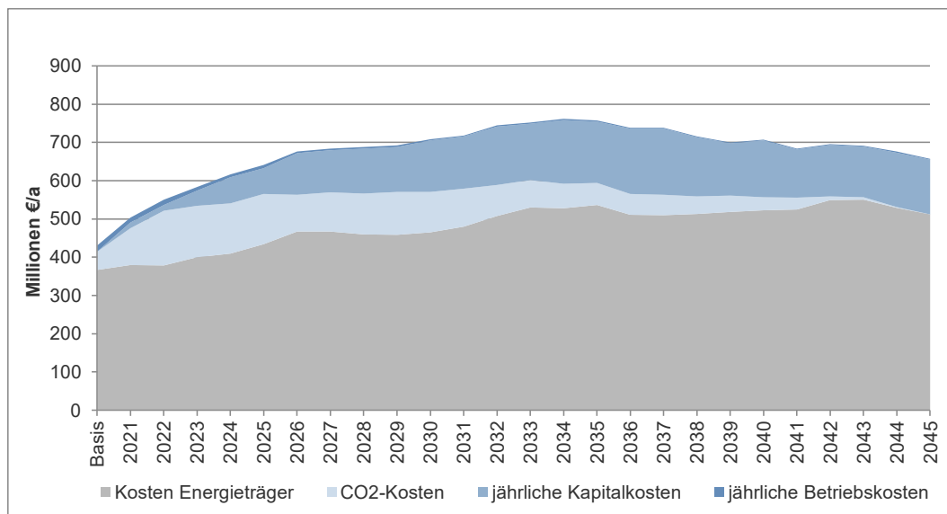
Abbildung 35: Entwicklung der energiebezogenen Kosten bis 2045 im Elektrifizierungspfad II (Pfad 3b)
