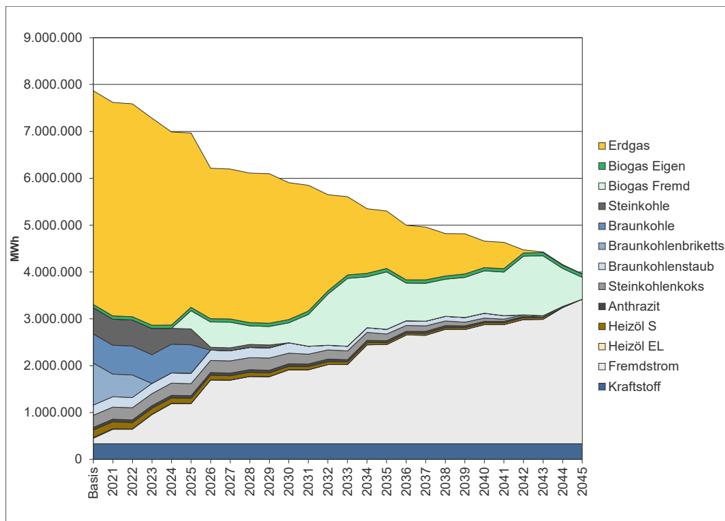
Abbildung 33: Entwicklung der energiebezogenen Kosten bis 2045 im Elektrifizierungspfad II (Pfad 3b)
