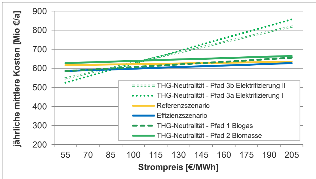
Abbildung 36: Sensitivitätsbetrachtung der mittleren jährlichen energiebezogenen Kosten abhängig vom Strombezugspreis
