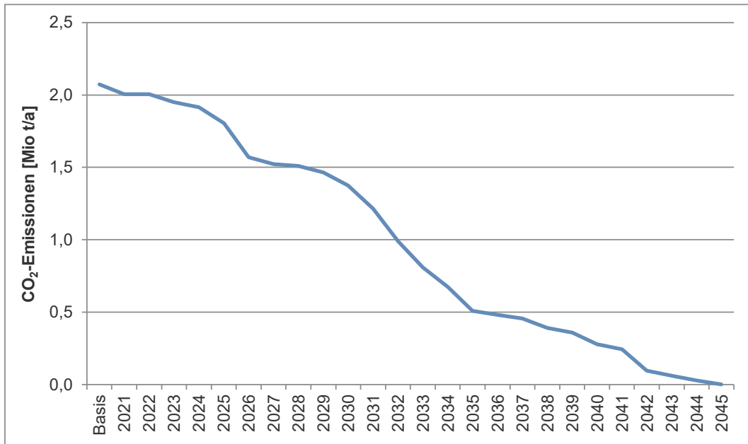
Abbildung 31: Entwicklung der CO 2 -Emissionen bis 2045 im Elektrifizierungspfad I (Pfad 3a)
