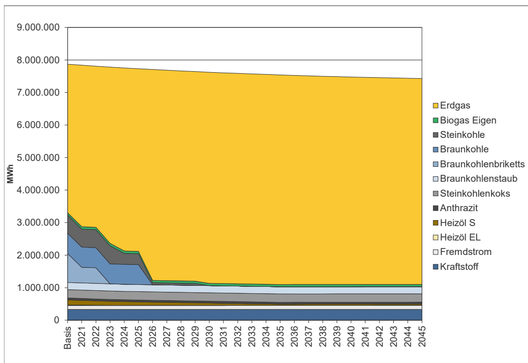
Abbildung 9: Entwicklung des Energieträgereinsatzes bis 2045 im Referenzszenario
