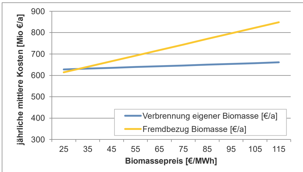
Abbildung 29: Sensitivitätsbetrachtung der mittleren jährlichen energiebezogenen Kosten abhängig von den Bezugskosten für Biomasse
