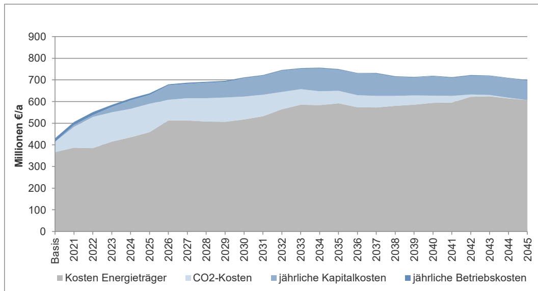
Abbildung 32: Entwicklung der energiebezogenen Kosten bis 2045 im Elektrifizierungspfad I (Pfad 3a)
