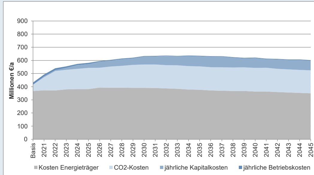
Entwicklung der jährlichen energiebezogenen Kosten bis 2045 im Effizienzscenario
