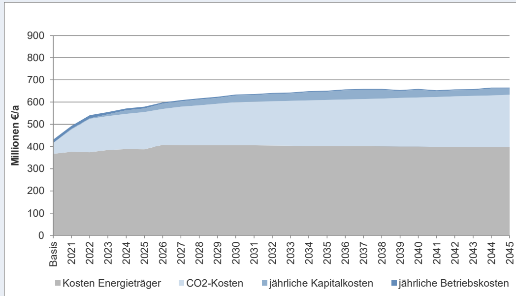
Entwicklung der jährlichen energiebezogenen Kosten bis 2045 im Referenzszenario
