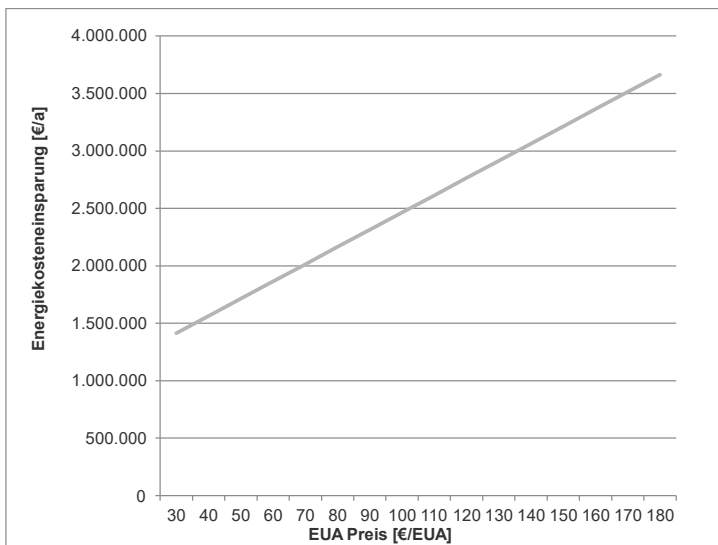
Abbildung 16: Energiekosteneinsparung einer exemplarischen Brüdenverdichtung in Abhängigkeit vom EUA-Preis
