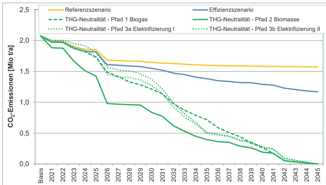
Abbildung 38: Entwicklung der CO 2 -Emissionen bis 2045 – Gegenüberstellung aller Szenarien
