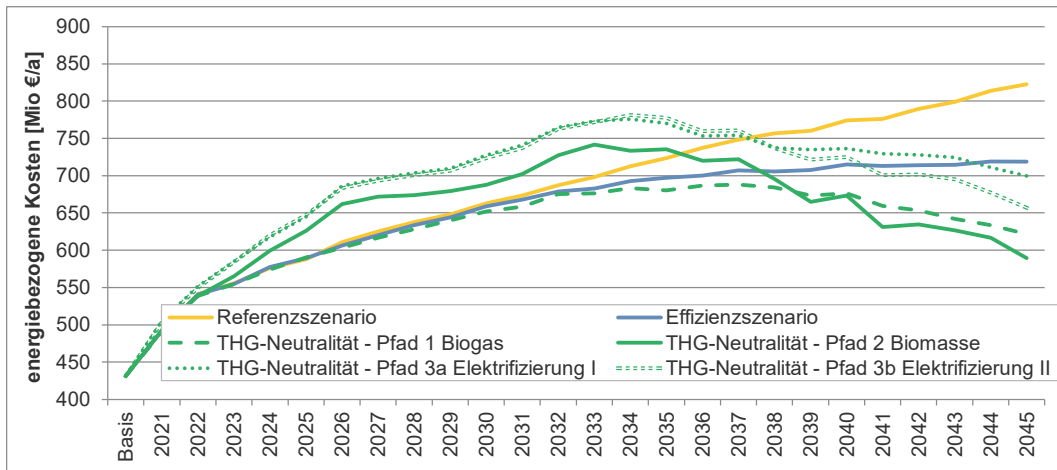
Abbildung 44 Energiebezogene Kosten aller Szenarien bei einem CO 2 -Preisfad bis 250 €/t im Jahr 2045
